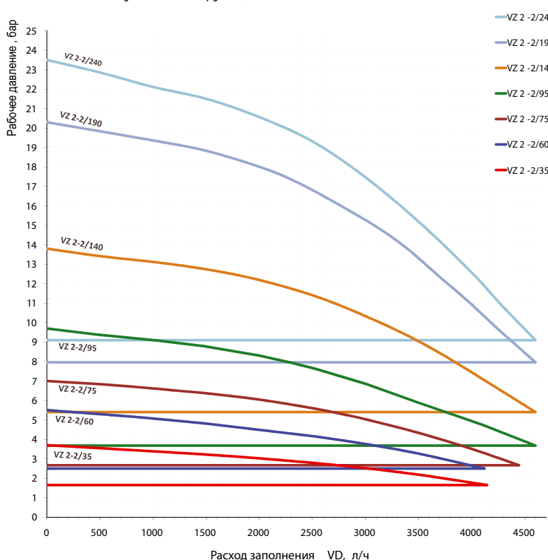
Насосные установки с функцией заполнения Variomat VZ
